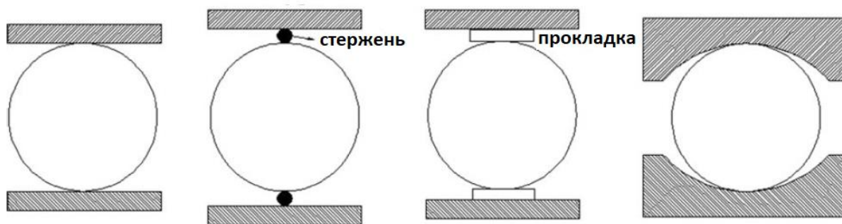
Рис. 1. Варианты передачи нагрузки при испытаниях цилиндрических образцов сжатием по образующим
