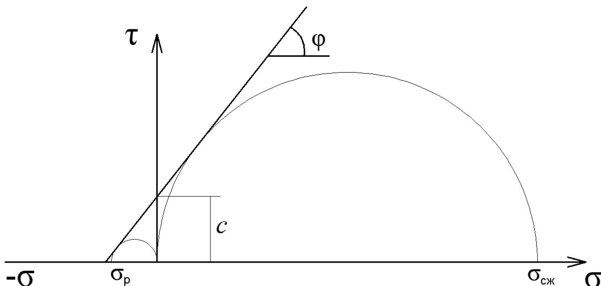
Рис. 2. Схема к определению параметров условия прочности Кулона-Мора для скального грунта
