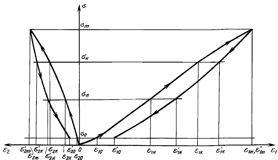
Рис. 1. Экспериментальные зависимости, полученные при одноосном сжатии скального грунта
