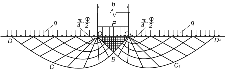
Рис. 1.4. Расчетная схема определения несущей способности основания центрально нагруженного фундамента
