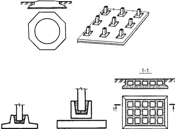
Конструкции фундаментов, грунты оснований которых работают в условиях пространственной деформации
