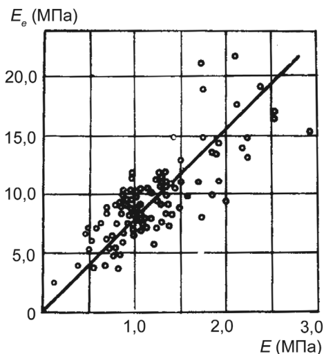
Рис. 1.3. Зависимость между модулем деформации и модулем упругости (Баркан Д.Д. и др., 1974)
