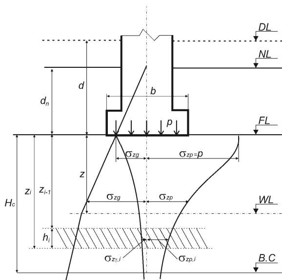
Рис. 1.1. Расчетная схема к определению осадки фундаментов
