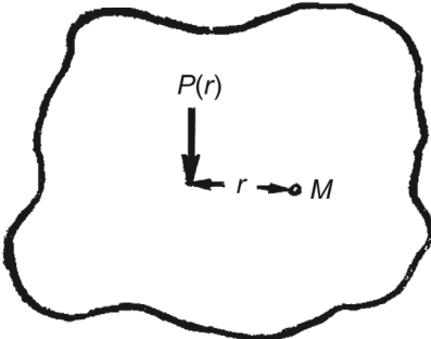
Задача Буссинеска
